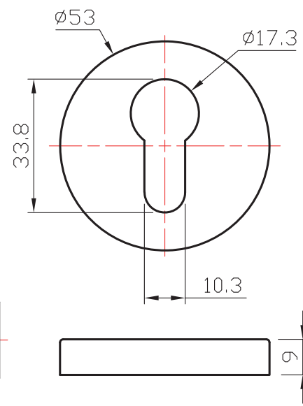
Bocacilindro
